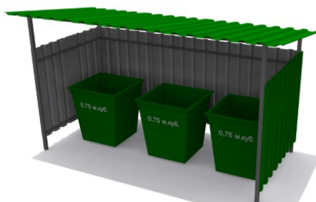
Площадка ТБО на 3 контейнера с навесом Размеры: 4000x1500x2000 мм. Цена: 85 800р.
