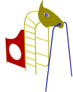
Спортивный элемент "Лаз-лошадка" №27 Размеры: 2500x1000x2000 мм. Возраст: 3-12 лет. Цена: 39 600р.
