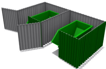
Площадка ТБО на 2 бункера-накопителя с воротами Размеры: 6000x4000x1700 мм. Цена: 223 300р.
