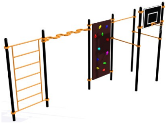
Воркаут-комплекс классический №61 Размеры: 5800x1600x3500 мм. Возраст: от 14 лет. Цена: 149 600р.
