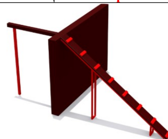
Спортивный элемент "Забор с наклонной доской" №21 Размеры: 4500x2500x2000 мм. Возраст: от 14 лет. Цена: 126 500р.
