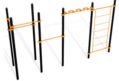
Воркаут-комплекс классический №30 Размеры: 6400x1400x2600 мм. Возраст: от 14 лет. Цена: 107 800р.
