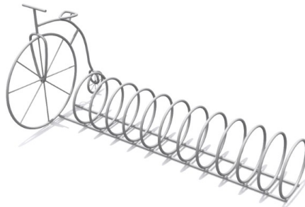
Велопарковка 10-ти местная "Классик" Размеры: 4000x800x1300 мм. Цена: 60 500р.
