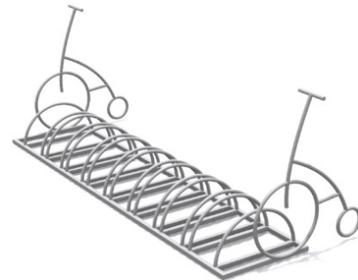
Велопарковка 10-ти местная "Марло" Размеры: 4000x800x1200 мм. Цена: 44 000р.
