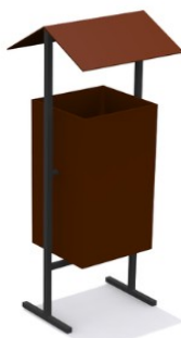
Урна ТБО 20 л. "Эконом" №5 Размеры: 250x250x600 мм. Цена: 6 600р.
