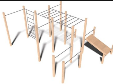
Воркаут-комплекс «ЭкоСпорт» №17 Размеры: 6300x4300x2500 мм. Возраст: от 14 лет. Цена: 242 000р.
