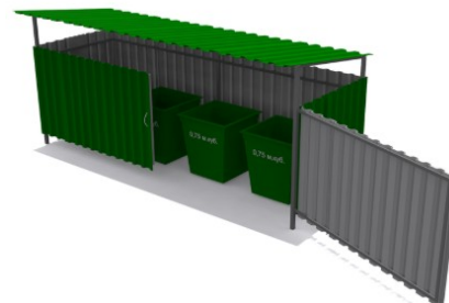
Площадка ТБО на 4 контейнера с навесом и воротами Размеры: 5200x1500x2000 мм. Цена: 151 800р.
