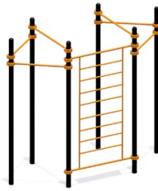
Воркаут-комплекс классический №26 Размеры: 4000x1400x2600 мм. Возраст: от 14 лет. Цена: 90 200р.
