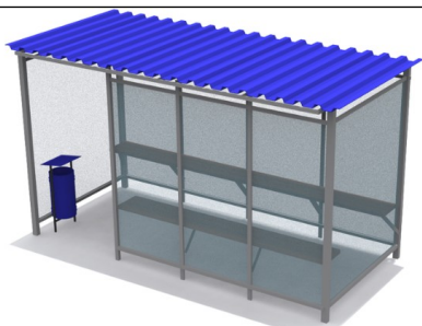
Павильон для курения "Европа" Размеры: 3500x2000x2400 мм. Цена: 313 500р.
