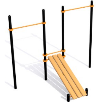
Воркаут-комплекс классический №33 Размеры: 3200x1600x2600 мм. Возраст: от 14 лет. Цена: 68 200р.
