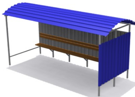
Остановочный павильон "Стандарт" Размеры: 5000x2000x2400 мм. Цена: 187 000р.
