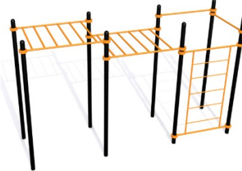
Воркаут-комплекс классический №29 Размеры: 5200x1400x2600 мм. Возраст: от 14 лет. Цена: 123 200р.
