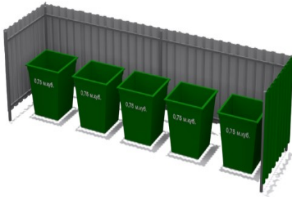
Площадка ТБО на 5 контейнеров Размеры: 6400x1500x1500 мм. Цена: 92 400р.
