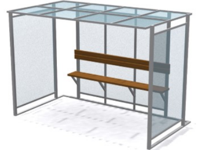
Остановочный павильон "Кубань" Размеры: 3500x2000x2500 мм. Цена: 291 500р.
