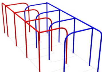
Спортивный элемент "Лабиринт" №34 Размеры: 3200x1500x1000 мм. Возраст: 3-12 лет. Цена: 34 100р.
