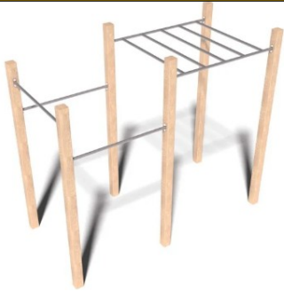
Воркаут-комплекс «ЭкоСпорт» №13 Размеры: 3000x1400x2500 мм. Возраст: от 14 лет. Цена: 78 100р.
