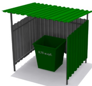
Площадка ТБО на 1 контейнер с навесом Размеры: 1700x1500x2000 мм. Цена: 50 600р.
