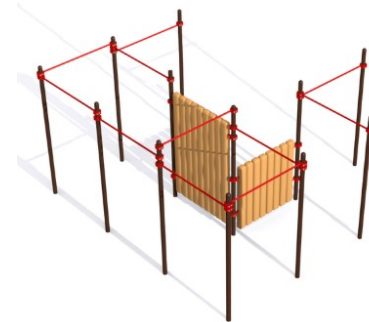
Воркаут-комплекс для паркура №7 Размеры: 4500x4500x2600 мм. Возраст: от 14 лет. Цена: 195 800р.
