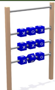
Игровая панель "Крестики-нолики" Размеры: 1000x100x1300 мм. Возраст: 3-7 лет. Цена: 28 600р.
