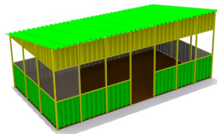
Теневой навес 40 м2 №3 Размеры: 8000х5000х2400 мм. Возраст: 3-14 лет. Цена: 671 000р.
