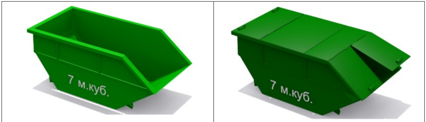
Бункер-накопитель ТБО 7 м3 Размеры: 3150x1850x1280 мм.
