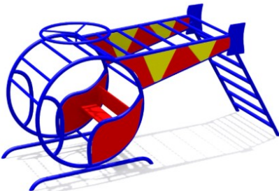
Спортивный элемент "Лаз- вертолет" №31 Размеры: 3000x1000x1600 мм. Возраст: 3-12 лет. Цена: 67 100р.
