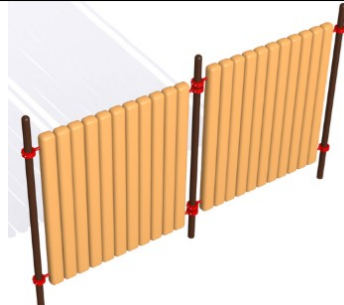
Воркаут-комплекс для паркура №11 Размеры: 3000x90x2600 мм. Возраст: от 14 лет. Цена: 103 400р.
