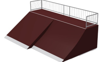
Рампа №21 Размеры: 7300х3500х2700 мм. Возраст: от 12 лет. Цена: 605 000р.
