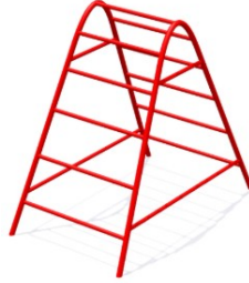
Спортивный элемент "Лаз-пирамида" №14 Размеры: 1500x1000x1100 мм. Возраст: 3-12 лет. Цена: 23 100р.
