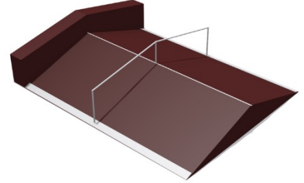
Рампа №15 Размеры: 5400х5000х1100 мм. Возраст: от 12 лет. Цена: 641 300р.
