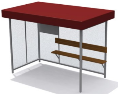
Остановочный павильон "Армада" Размеры: 3500x2000x2500 мм. Цена: 313 500р.
