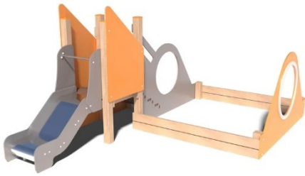
Игровой комплекс "ЭкоИгра" №11 Размеры: 3800х2600х1600 мм. Возраст: 3-7 лет. Цена: 199 100р.
