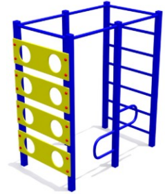
Спортивный комплекс №21 Размеры: 1700x800x2600 мм. Возраст: 6-14 лет. Цена: 59 400р.
