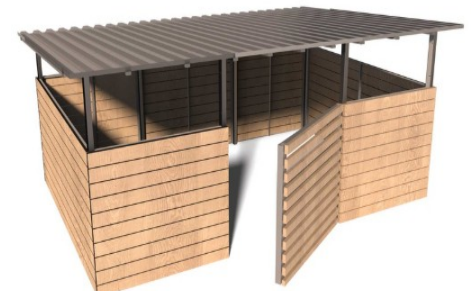
Контейнерная площадка "Евро" на 7 евроконтейнеров Размеры: 3500x2500x2400 мм. Цена: 363 000р.
