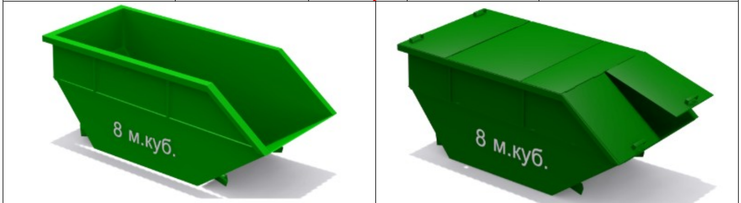
Бункер-накопитель ТБО 8 м3 Размеры: 3300x1900x1420 мм.
