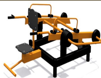
Тренажер силовой "Трицепс" Размеры: 2300x1600x1000 мм. Возраст: от 14 лет. Цена: 145 200р.
