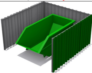
Площадка ТБО на 1 бункер-накопитель Размеры: 3000x4000x1700 мм. Цена: 94 600р.
