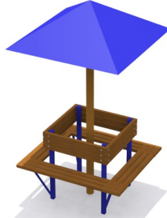
Пляжный зонт со скамейкой Размеры: 1200x1200x2300 мм. Цена: 53 900р.
