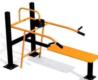
Тренажер силовой "Жим горизонтальный" Размеры: 2200x1100x1300 мм. Возраст: от 14 лет. Цена: 108 900р.
