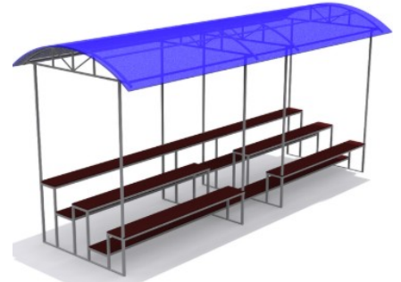
Трибуна 3-х рядная (32 места) №3 Размеры: 6500x2200x2800 мм. Цена: 269 500р.
