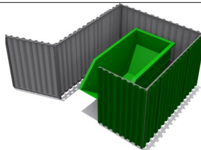
Площадка ТБО на 1 бункер-накопитель с воротами Размеры: 3000x4000x1700 мм. Цена: 122 100р.
