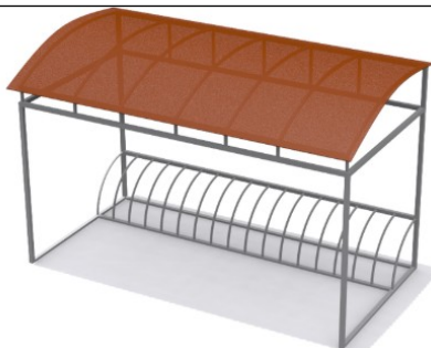
Велопарковка 16-ти местная "Макси" Размеры: 3000x1600x2100 мм. Цена: 104 500р.
