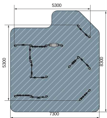
план, зона безопасности
