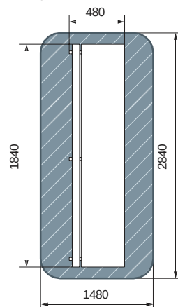
план, зона безопасности
