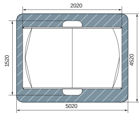
план, зона безопасности
