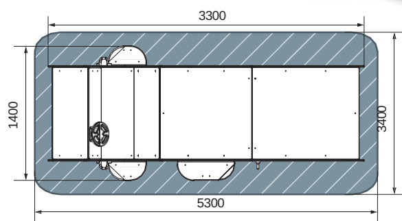
план, зона безопасности
