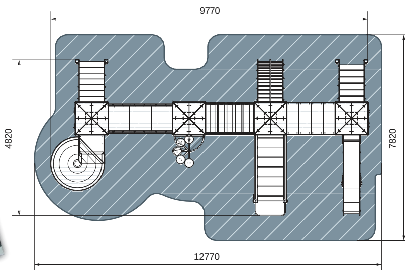
план, зона безопасности
