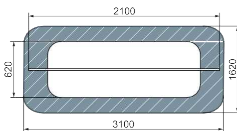
план, зона безопасности
