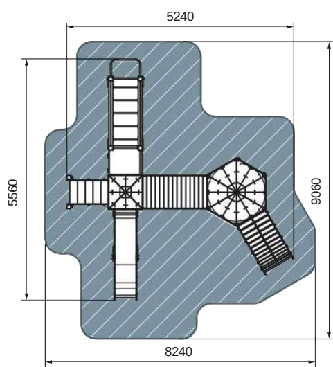
план, зона безопасности
