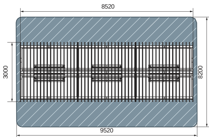
план, зона безопасности
