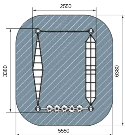
план, зона безопасности
