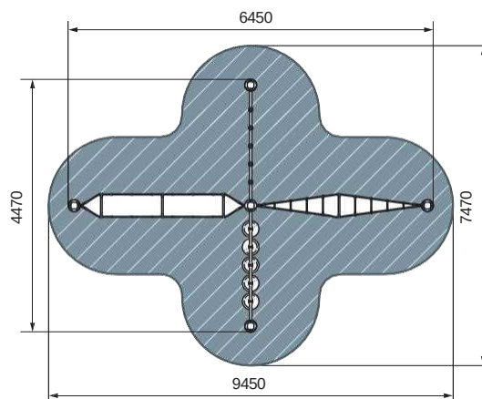
план, зона безопасности
