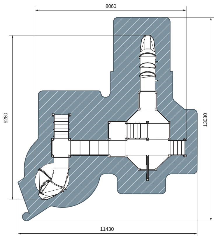
план, зона безопасности
